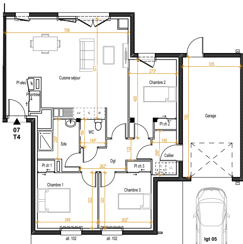
Plan rez-de-chaussée
