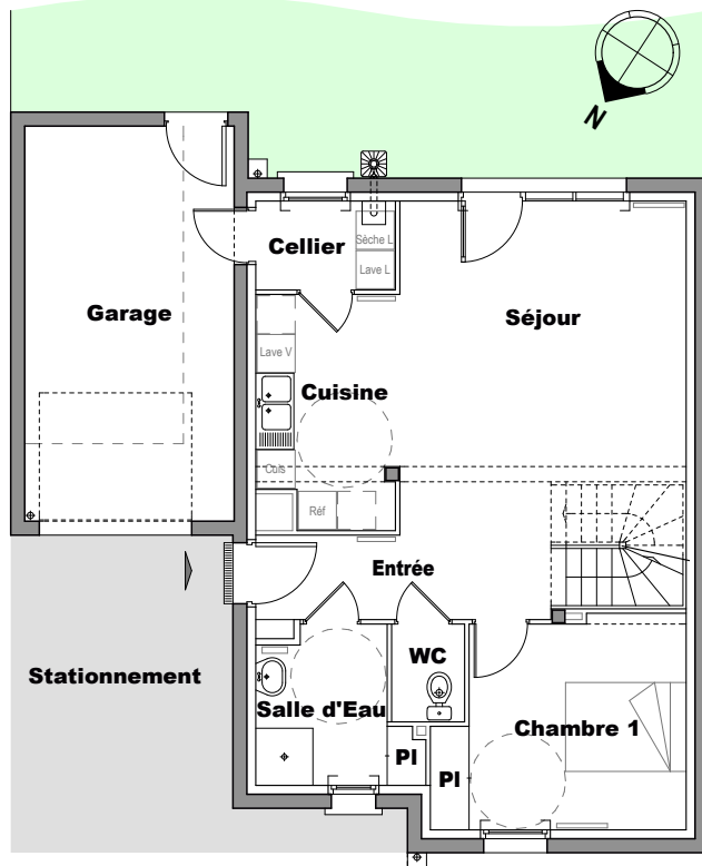
▼ Plan rez-de-chaussée
